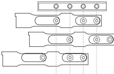
Posición 1: 3 tornillos
